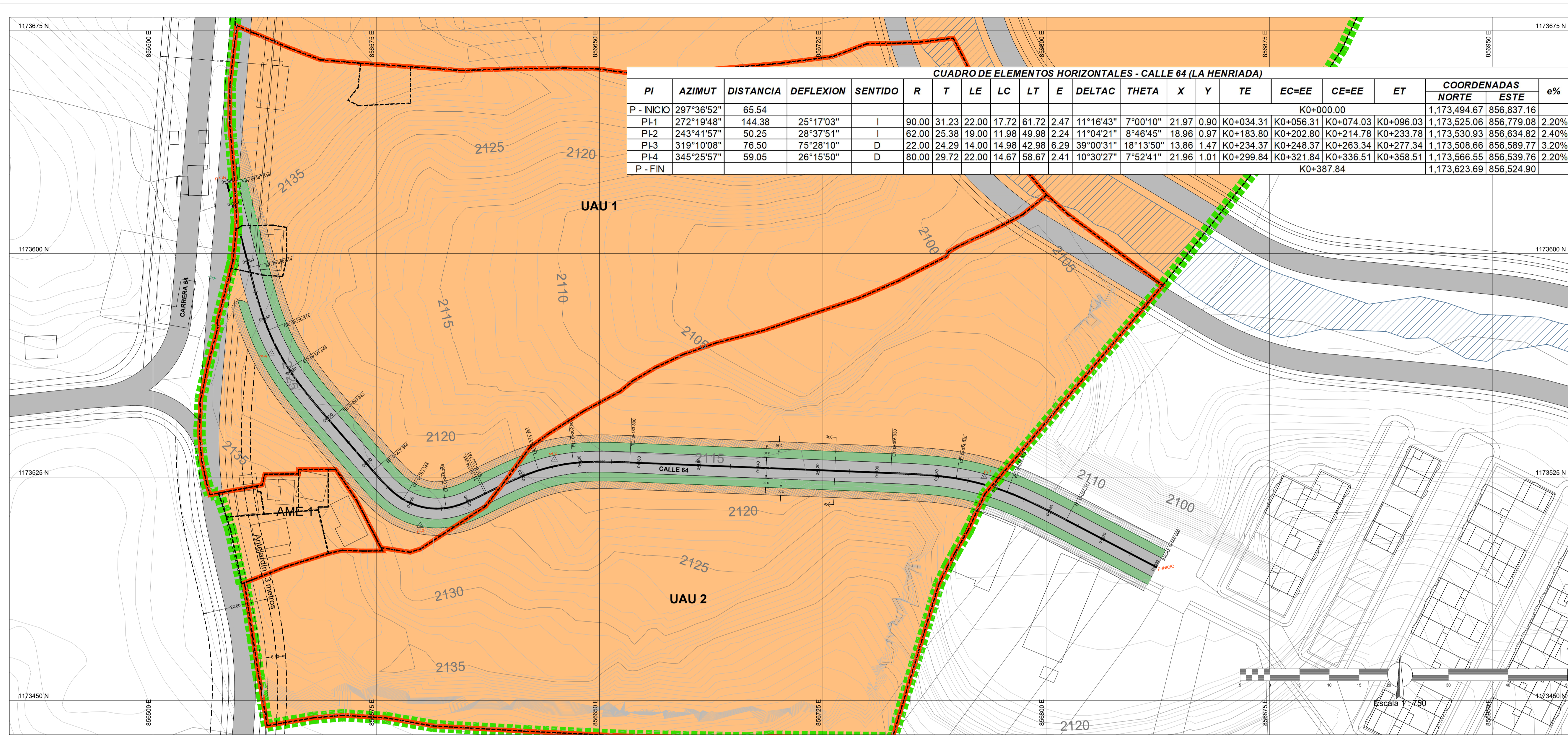
PLANTA CALLE 64 ENTRE MIRADOR DEL LAGO Y CARRERA 54 (FONTIBÓN) ESCALA 1:750
